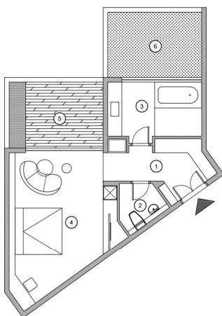
PHÒNG LOẠI C - 78M2
