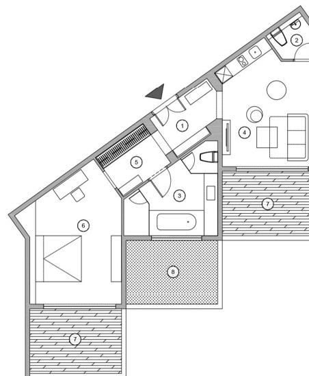
PHÒNG LOẠI D - 118M2
